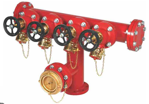
4 - Way Stand Post SPH-4W
