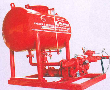
Foam Skid (Tank - 800 Ltr.)
